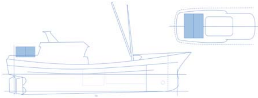
Afbeelding 10: LNG-opslag bovendeks.
