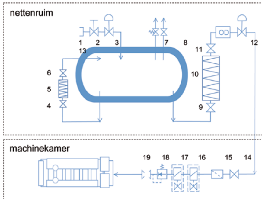
Afbeelding 14: Schematische weergave gastoevoersysteem koter AG-1.
