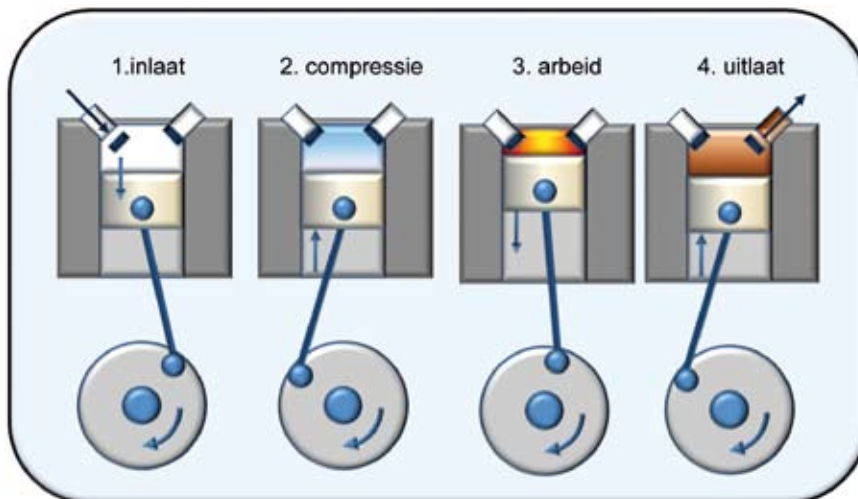
Afbeelding 3: Schematische voorstelling viertaktdieselmotor.
